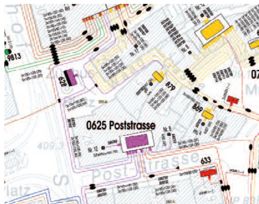
Ausschnitt aus einem Netzplan.
